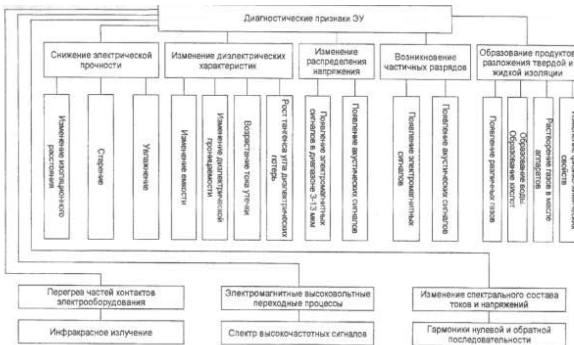
Рисунок 1. Блок-схема признаков дефектов в электроустановках
