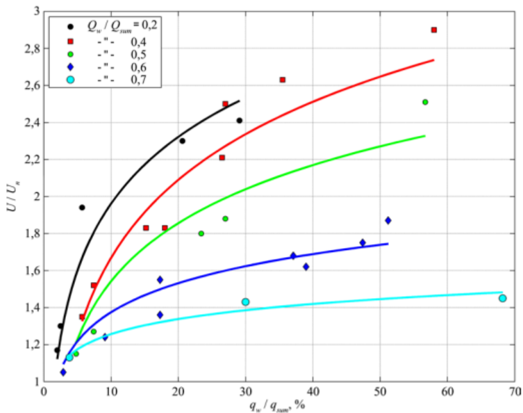
Рис. 1. График определения количества твердого стока, захватываемого в канал фронтального водозабора
